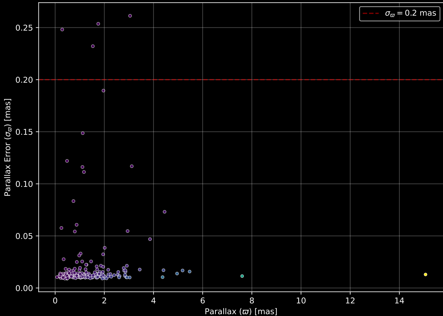
GALAH DR4 Field: [2884] Parallax Quality (n= 261)
