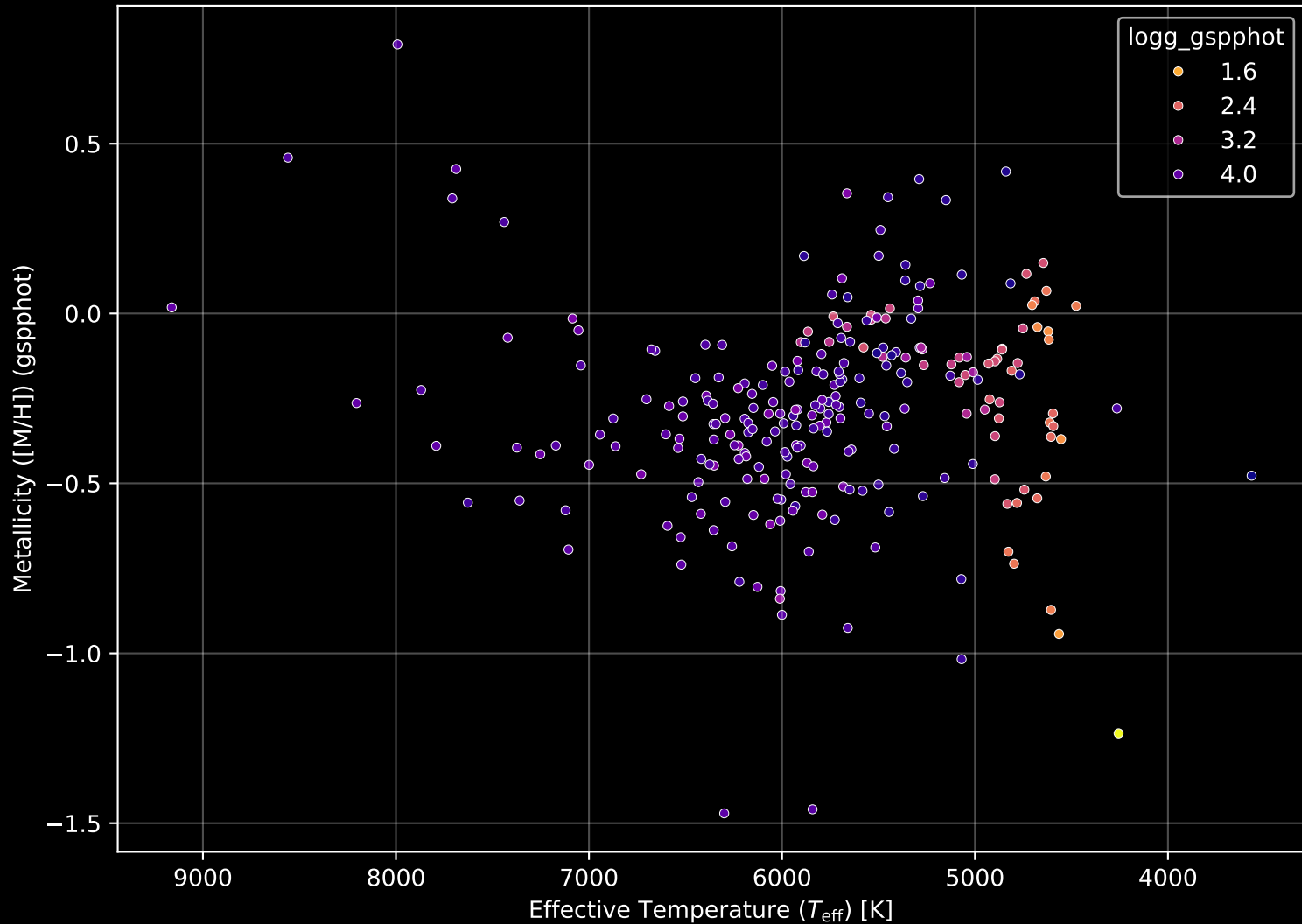
GALAH DR4 Field: [2884] Stellar Population Parameters (n= 261)
