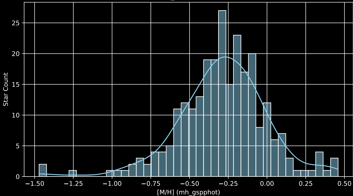
GALAH DR4 Field: [2884] [M/H] (mh_gspphot) (n= 260)
