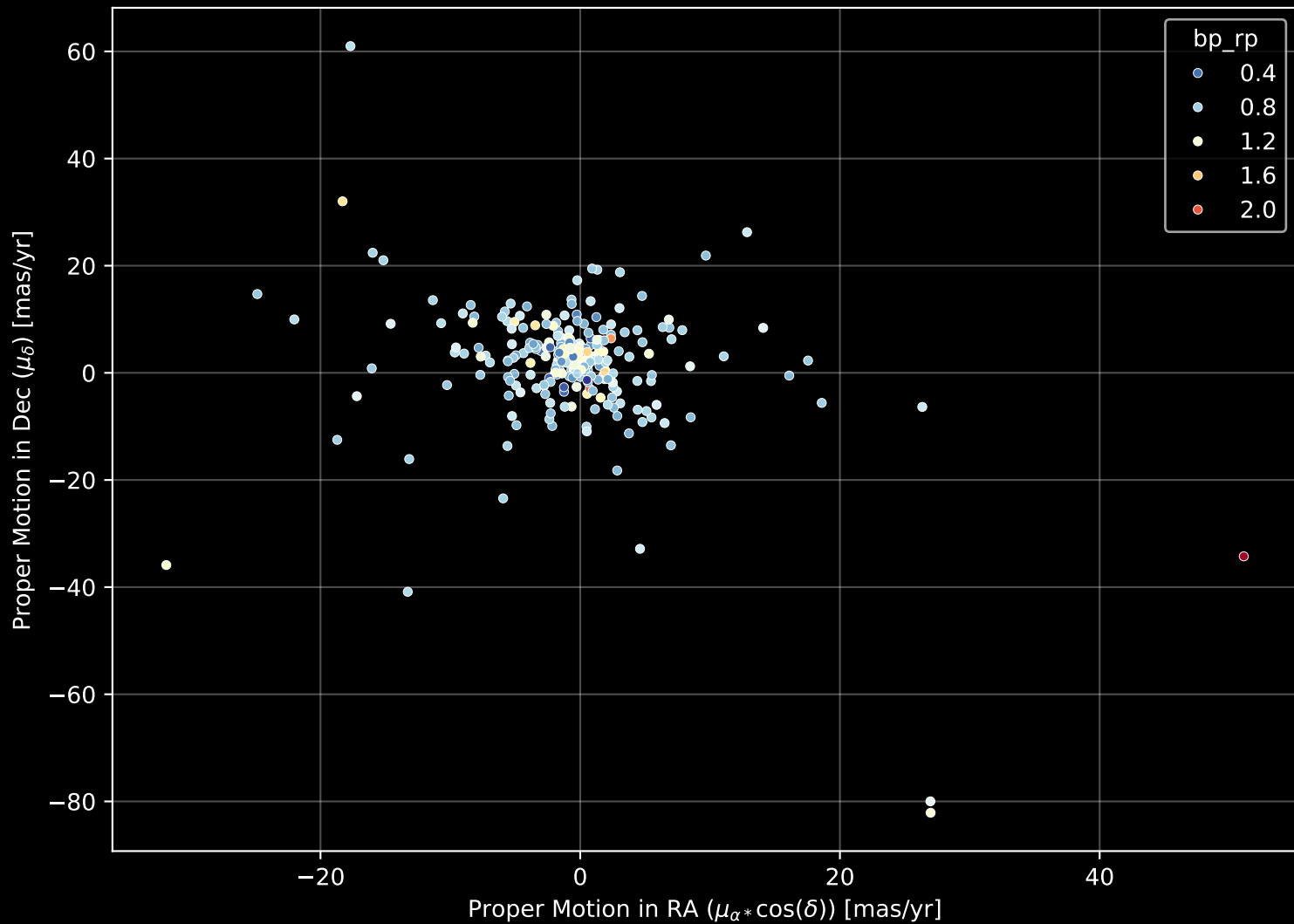
GALAH DR4 Field: [2884] Proper Motion Diagram (n= 261)
