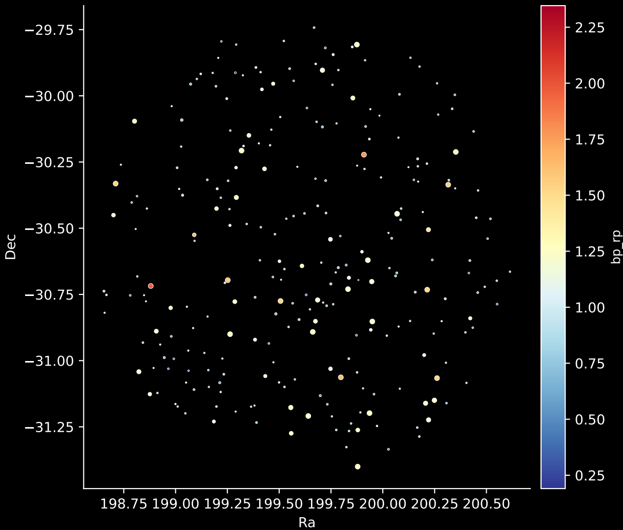
GALAH DR4 Field: [2884] Stars: 261
